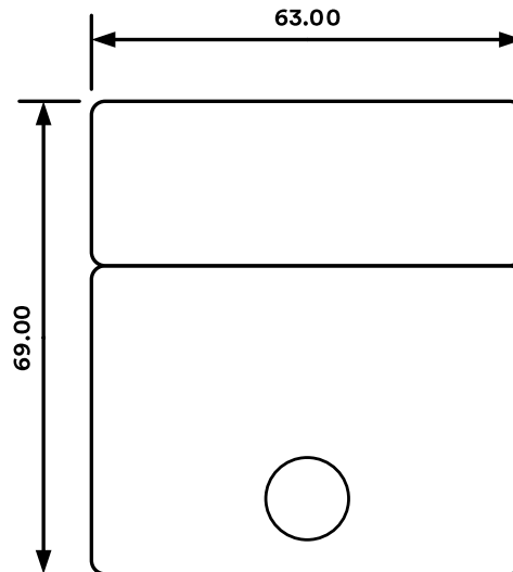
Abmessungen [mm] Einzelgehäuse und Leuchteneinsatz
